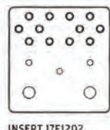
INSERT 17F12Q2 (12) SIZE 16 FIBRE OPTIC (3) SIZE 16 (2) SIZE 8 QUADRAX
